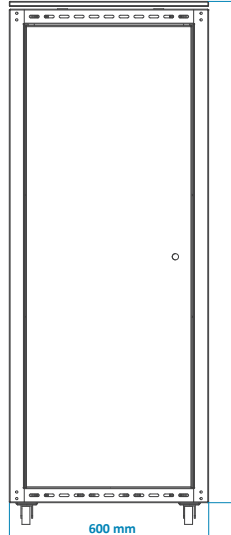
ARKA GÖRÜNÜM
