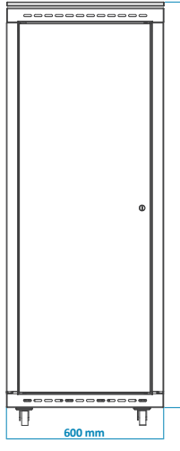
ARKA GÖRÜNÜM
