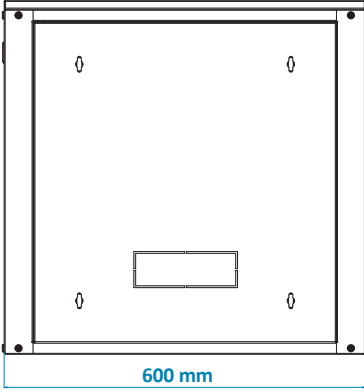
ARKA GÖRÜNÜM
